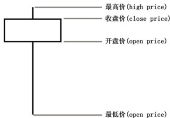
图4-1 Pinbar示例
